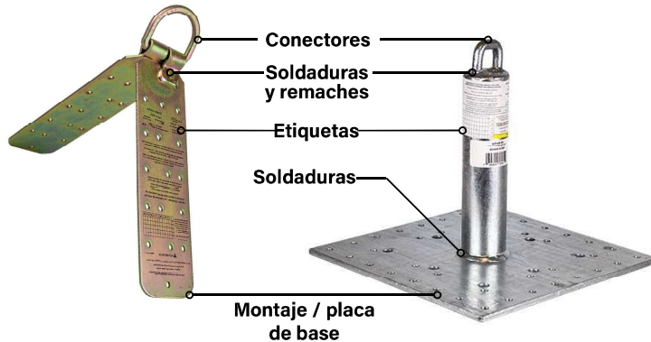
Anclaje de temple
