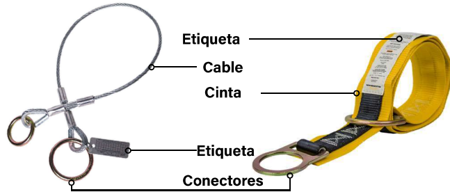
Anclaje para eslinga de cable
